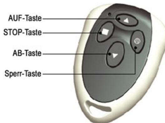
1-Kanal Minisender
